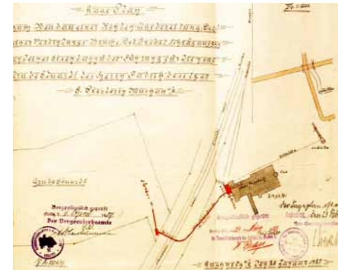
Übersichtsplan der Ziegelei Tiesler mit Brückenbauwerk 1927. (3)
